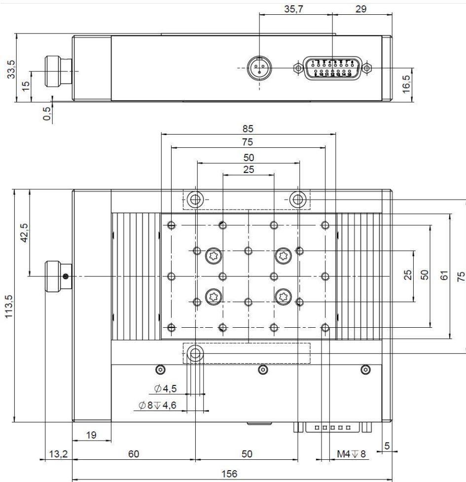
M-605.1DD, 尺寸单位为毫米
